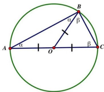
图 7：泰勒斯定理
